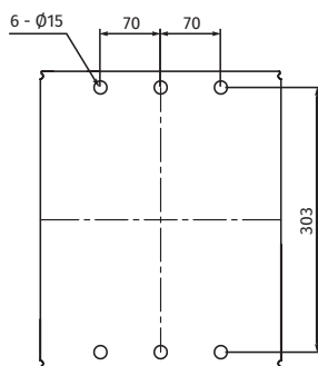
4 полюса
