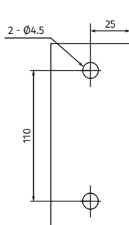
2 полюса
