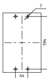
Размеры установки на щите 3 полюса
