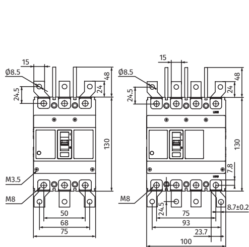
3 полюса
