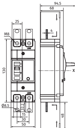
2 полюса
