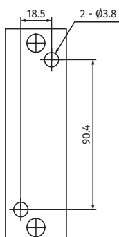
1 полюс
